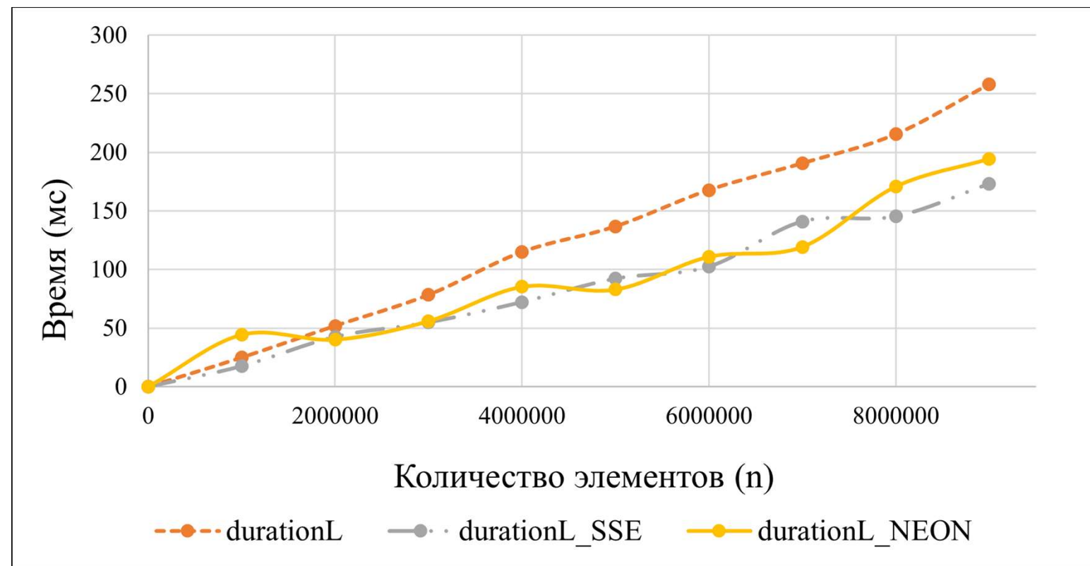
Рисунок 1 – График сравнений производительности алгоритма Левенштейна
